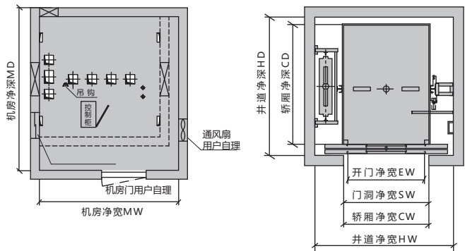
机房平面图
