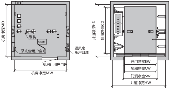
机房平面图
