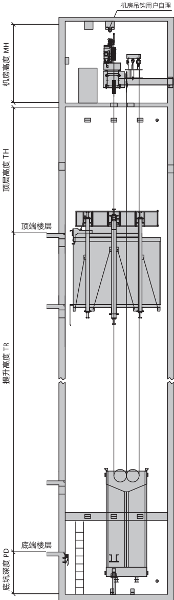
井道立面图
