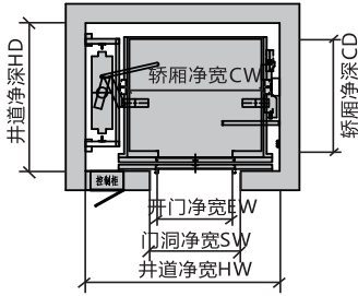
井道平面图 Shaft Plane
