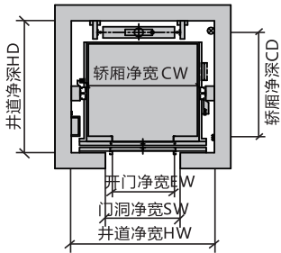
井道平面图 Shaft Plane
